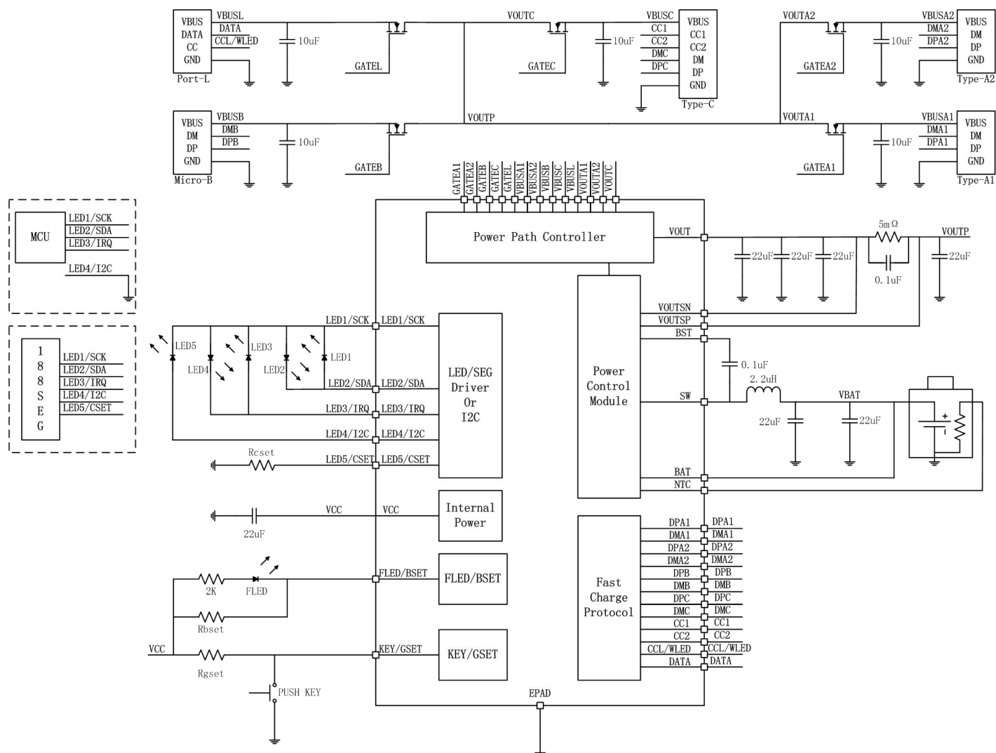
4. 功能框图
